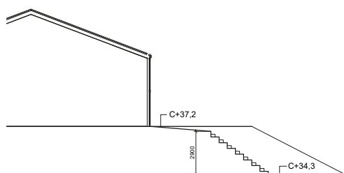
SNITT NY TRAPP/ SITTETRAPP
