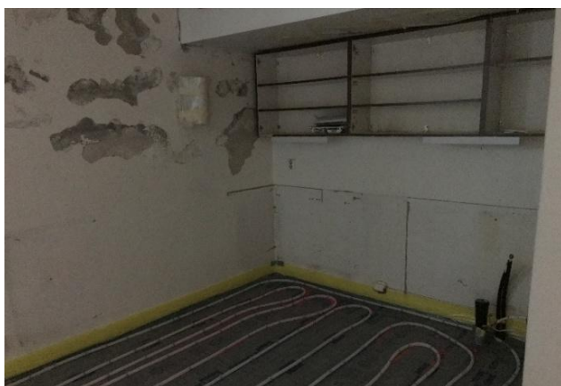
Vannledningene fra de 400 m dype energibrønnene som ble boret i jan-25 føres inn i maskinrommet.
